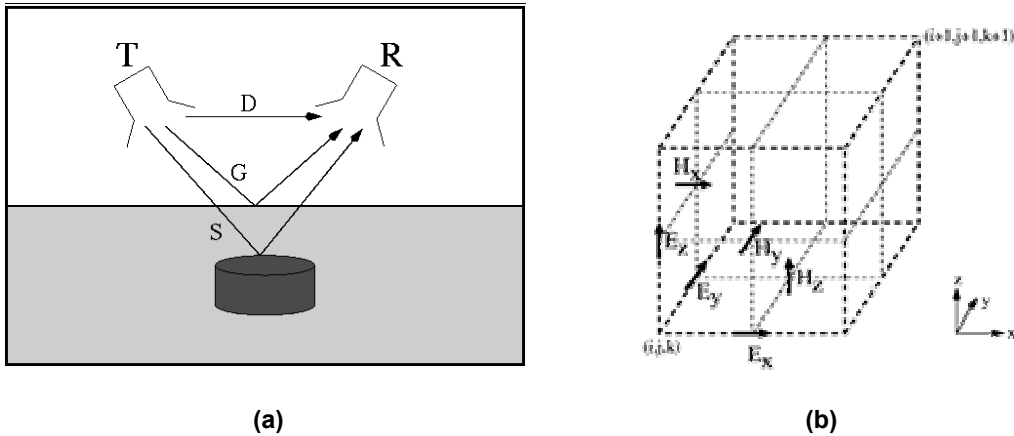
Şekil 1. Örnek bir GPR problemi ve Yee hücresi.
