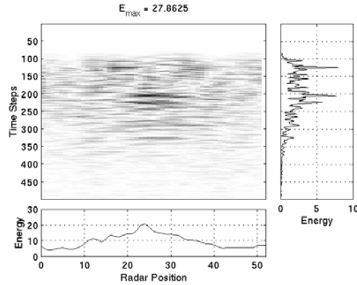
Şekil 7. İkinci heterojen toprak modeliyle elde edilmiş plastik mayın benzetimi sonuçları.
