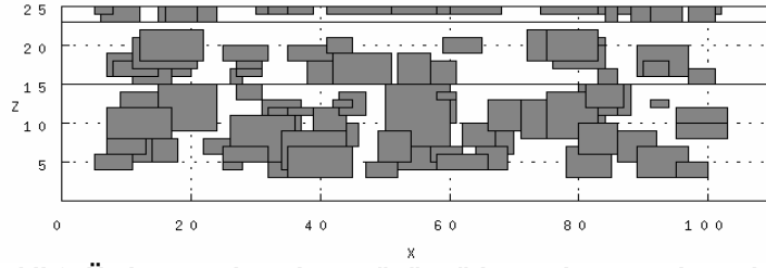
Şekil 8. Üç katmandan oluşan üçüncü heterojen toprak modeli.
