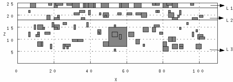
Şekil 4. Üç katmandan oluşan birinci heterojen toprak modeli.
