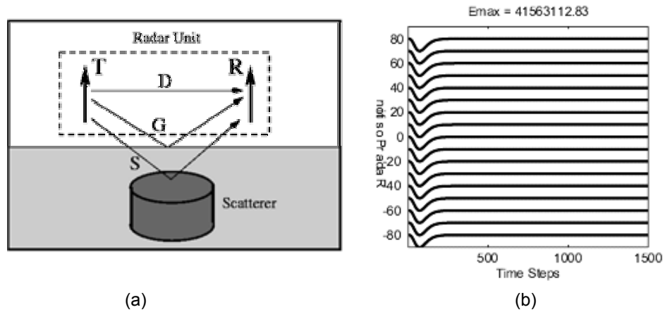
Şekil 2. Verici alıcı konfigürasyonu ve 25 cm derine gömülü iletken cismin benzetim sonuçları.
