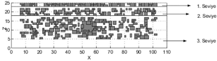
Şekil 6. Üç katmandan oluşan ikinci heterojen toprak modeli.
