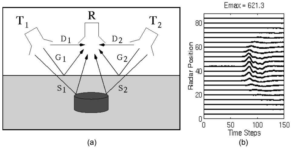
Şekil 10. İki vericili GPR modeli ve 2.5 cm derine gömülü iletken cismin benzetim sonuçları.
