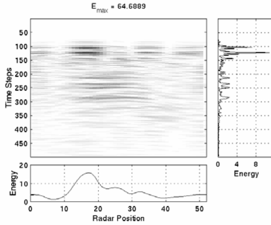
Şekil 9. Üçüncü heterojen toprak modeliyle elde edilmiş plastik mayın benzetimi sonuçları.
