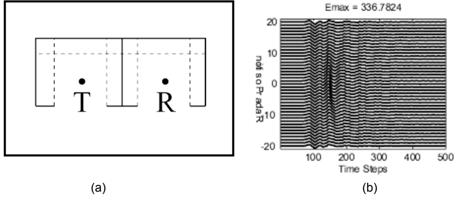
Şekil 3. Kalkanlı GPR modeli ve 2.5 cm derine gömülü iletken cismin benzetim sonuçları.
