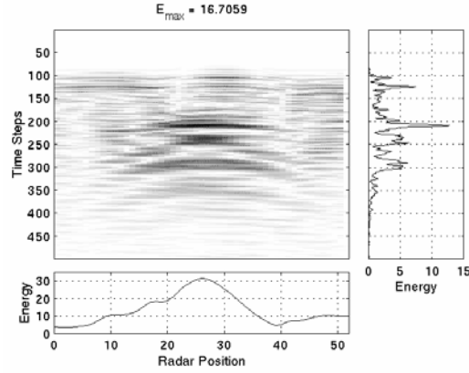
Şekil 5. Birinci heterojen toprak modeliyle elde edilmiş plastik mayın benzetimi sonuçları.
