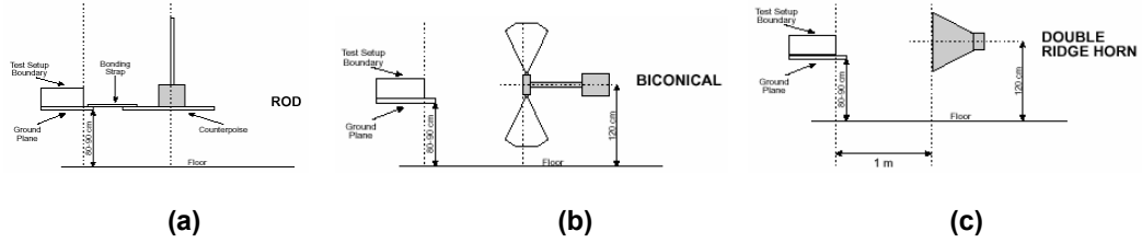
Şekil 4. MIL-STD-462'ye uygun olarak yaptığımız RE102 testlerinin anten konfigürasyonları.
